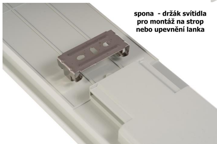
montáž spony krytu 2
